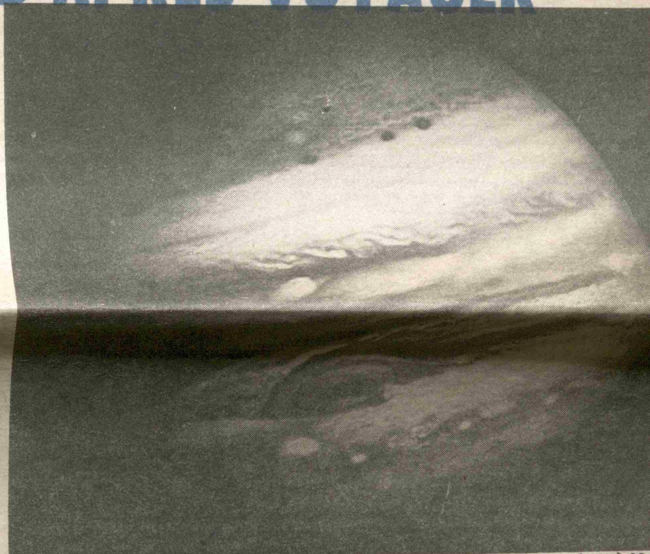
Jupiter par Voyager I, le 1er février 1979 alors que la sonde spatiale était à 32.7 millions de kilomètres. Des détails de 600 km de diamètres peuvent être résolus sur cette photo prise à travers un filtre bleu. (Photo de NASA)
